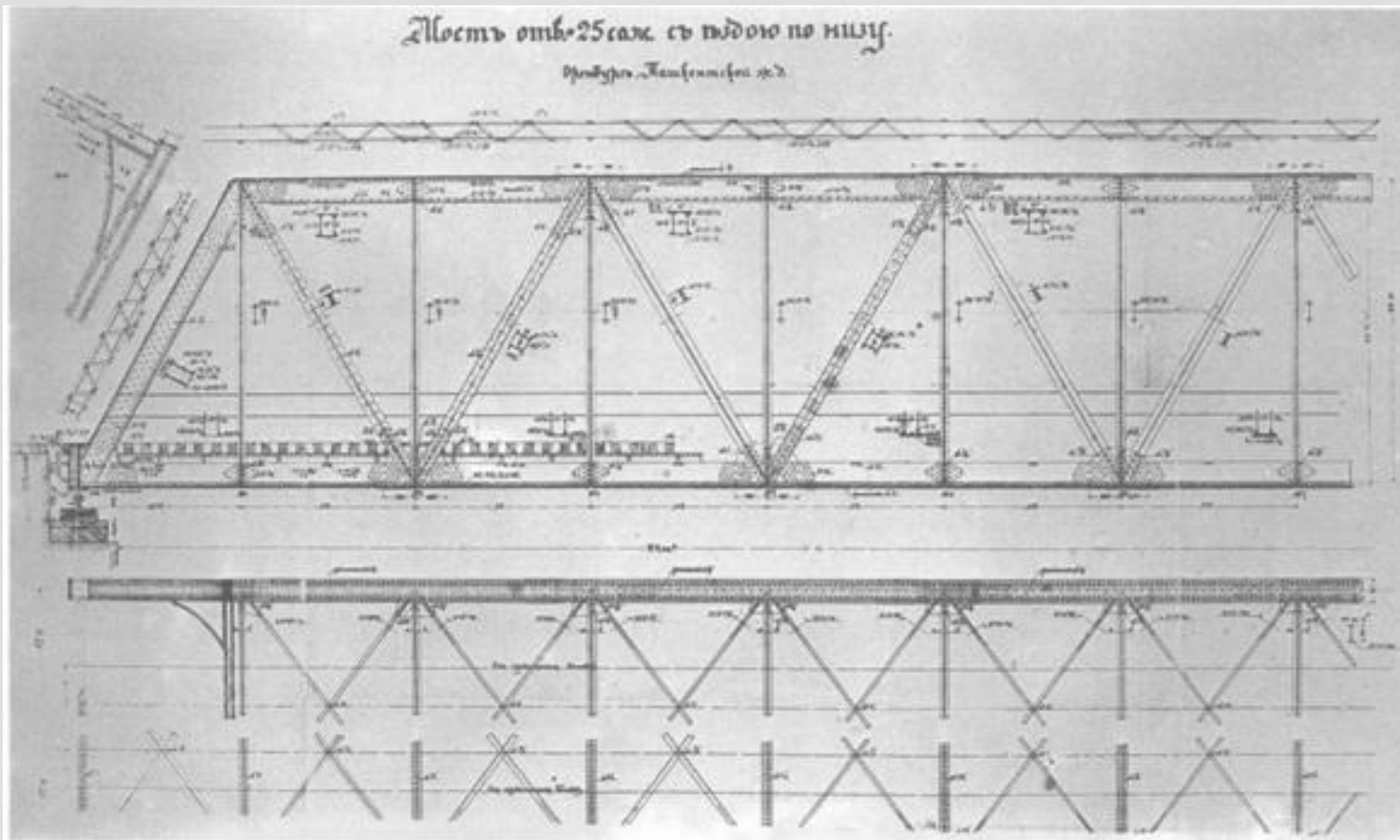
МОСТ ЖЕЛЕЗНОЙ ДОРОГИ ОРЕНБУРГ-ТАШКЕНТ. ПРОЛЕТ - 55 МЕТРОВ. РАБОЧИЙ ЧЕРТЕЖ.
