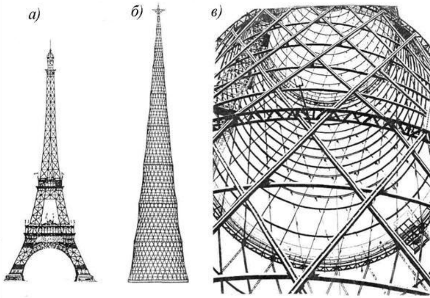
СРАВНЕНИЕ ВЫСОТ ЭЙФЕЛЕВОЙ БАШНИ (А) 1889Г. И ШАБОЛОВСКОЙ РАДИОБАШНИ (1919Г.) ПО ПЕРВОНАЧАЛЬНОМУ ПРОЕКТУ (Б); В - ФРАГМЕНТ РАДИОБАШНИ
