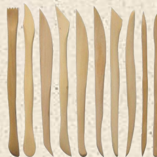
Стеки
