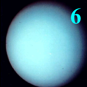
Уран
