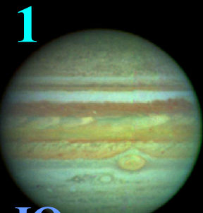
Юпитер
