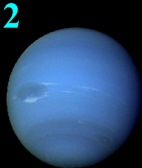
Нептун
