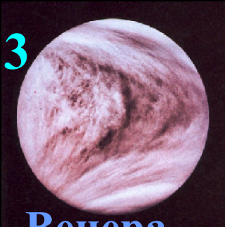
Венера
