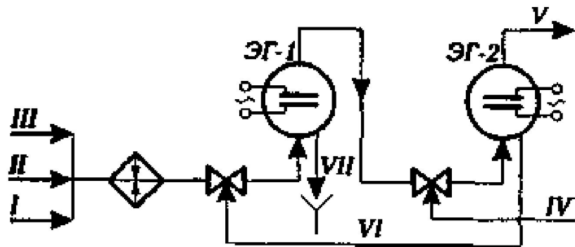
Рис. 5.3. Принципиальная схема установки (секции) электрообессоливания нефти: I—сырая нефть; II - деэмульгатор; III - содо-щелочной раствор; IV - свежая вода; VI - вода из электродегидратора 2-й ступени (ЭГ-2); VII -солёная вода из ЭГ-1.
