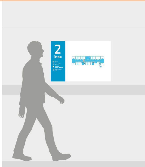
Схема этажа
