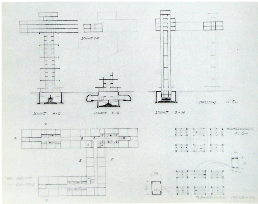
Рабочий чертеж №3. Конструктивный
