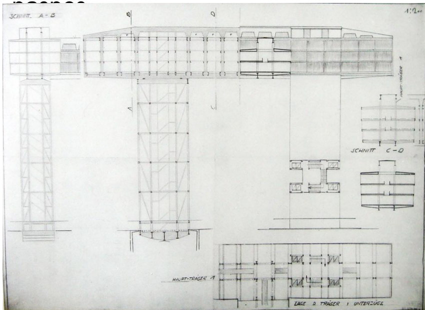
Рабочий чертеж №3. Конструктивный
