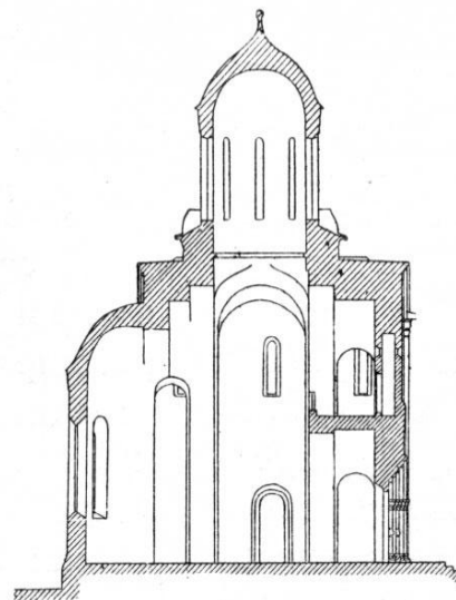
Продольный разрез
