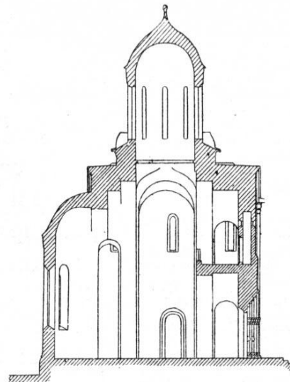
Продольный разрез
