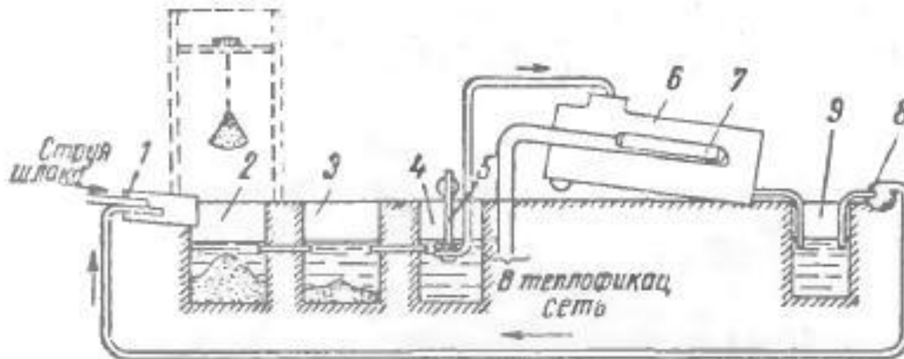
Рис. 5. Схема установки для использования тепла отвальных шлаков Красноуральского медеплавильного завода:
