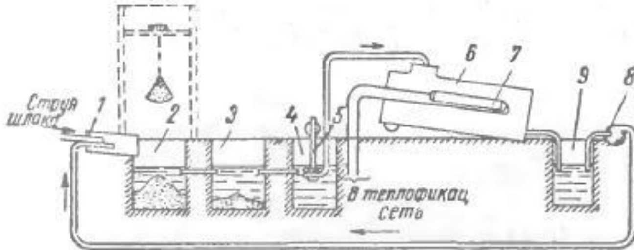
Рис. 5. Схема установки для использования тепла отвальных шлаков Красноуральского медеплавильного завода:
