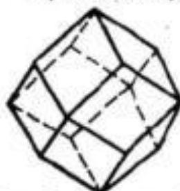
Ромбододекаэдр
