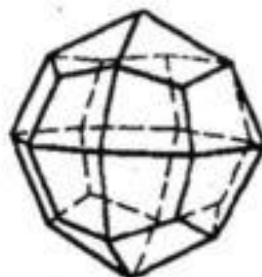
Тетрагон-триоктаэдр
