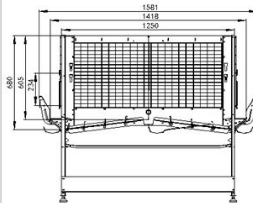
BH1250 鸡笼横断面
