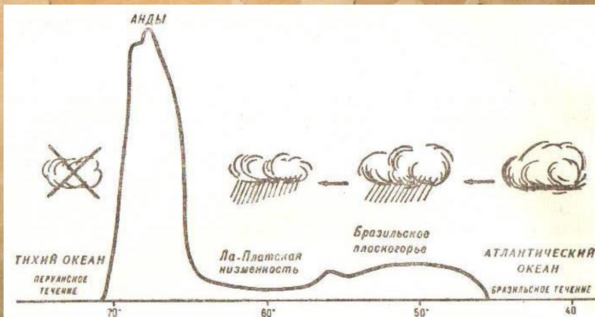
Рис. 30. Изменение климатических условий Южной Америки вдоль Южного тропика
