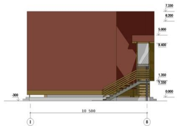
ФАСАД 1-8 М1:100
