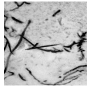
железобактерии
