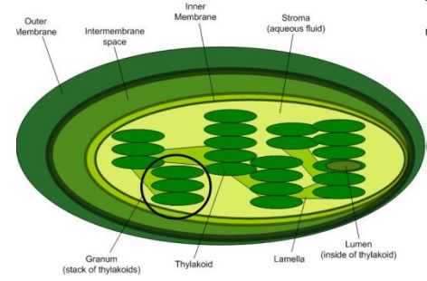
мембраны тилакоидов
