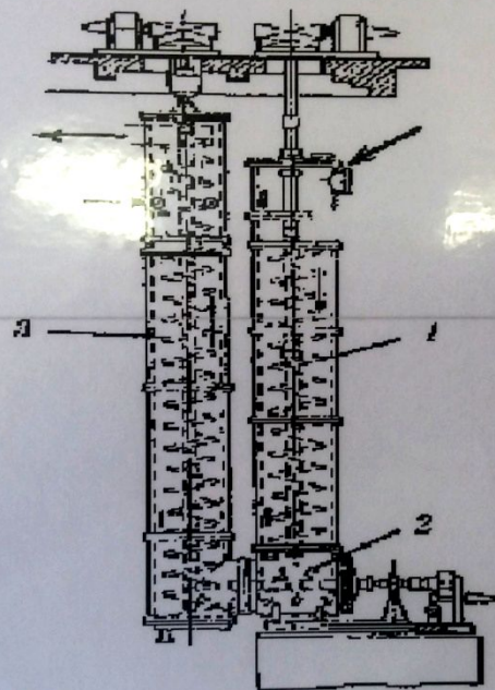
1-шикізат; 2-сорыт алғыш қондырғы; 3-шрот, экстрагент.
