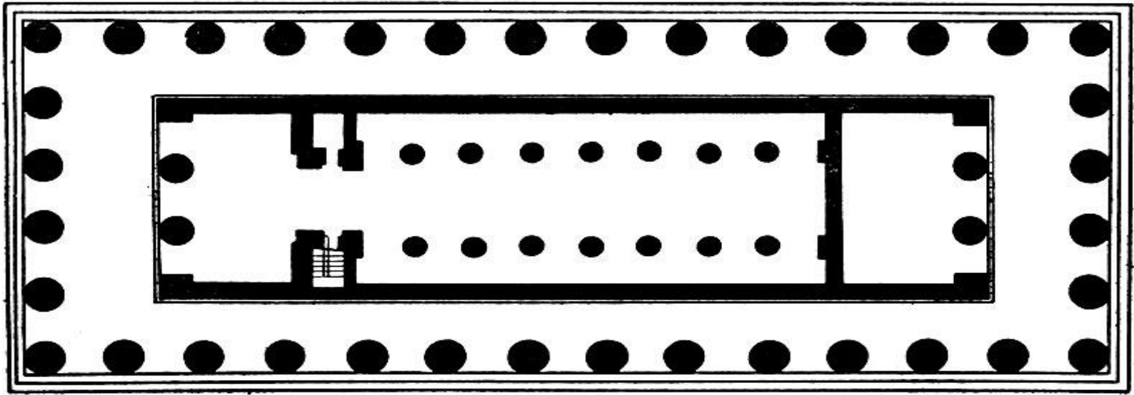
План храма Посейдона в Пестуме.
