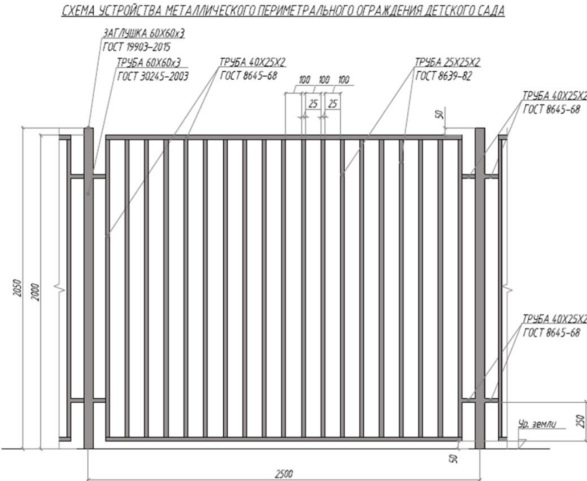
Ограждение металлическое (стандартный черный) – Палисад, h=2,0 м
