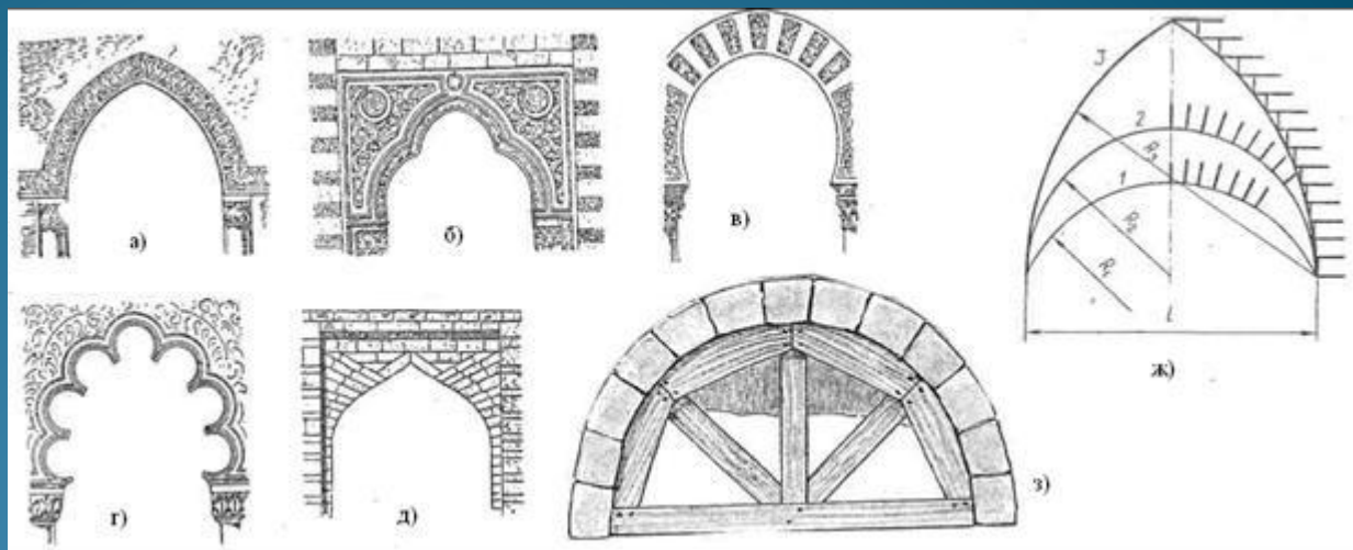
Арки Ислама: а - стрельчатая; б - трилистником; в - подковой; г - зубчатая; д - килевая; ж - очертания арок: 1 - пологой; 2 - полуциркульной; 3 - стрельчатой (ложной, безраспорной); з - деревянные распорки, которые придавали необходимую форму каменной кладке.
