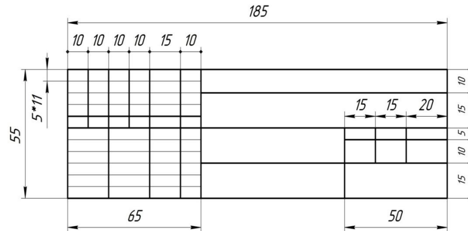
Основная надпись чертежа производственного здания
