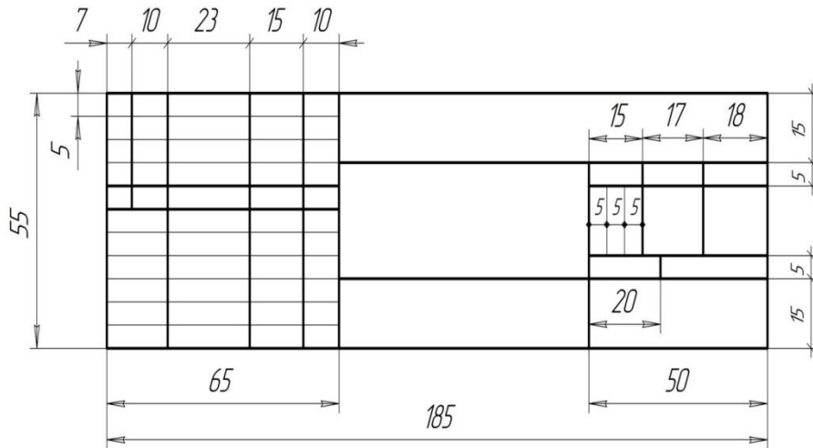
Образец заполнения основной надписи
