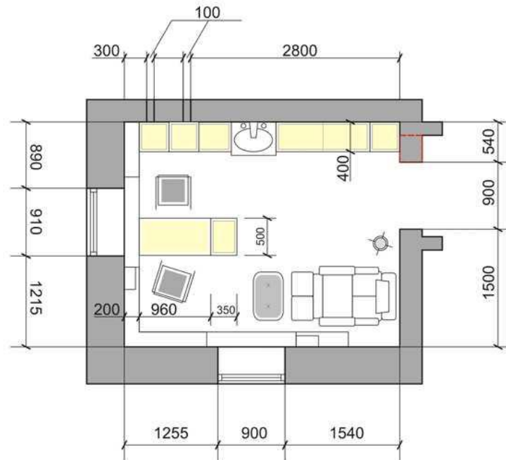
План расстановки мебели М 1:50
