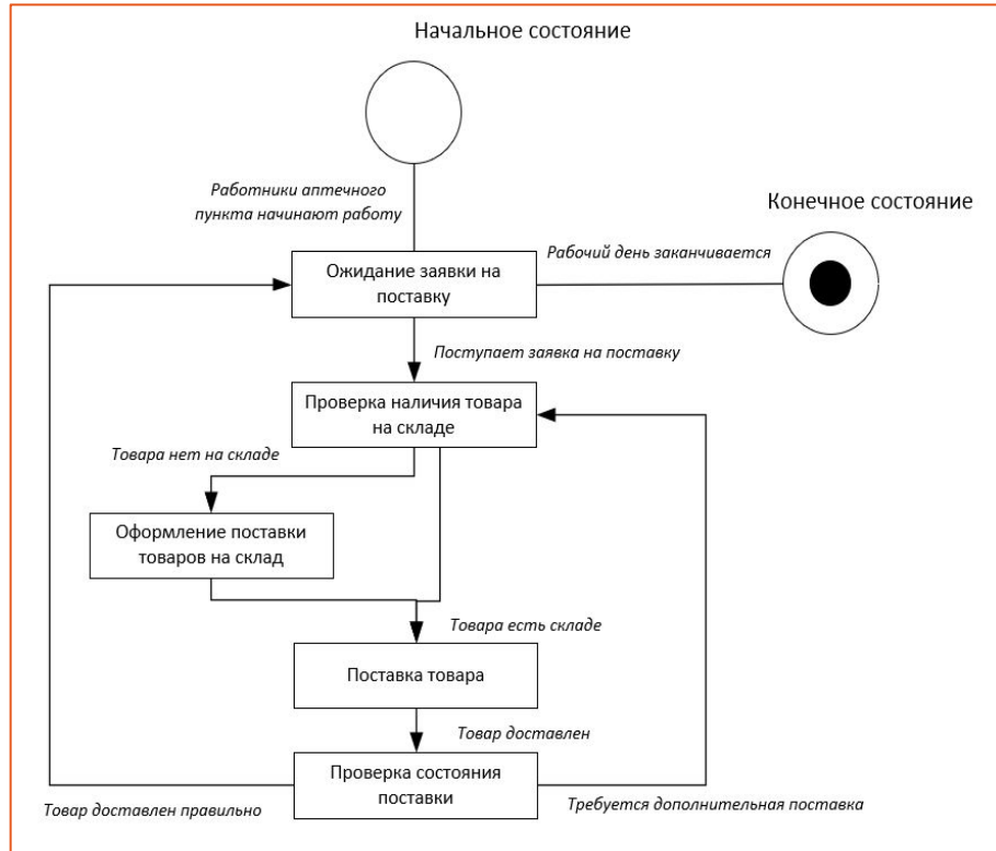
STD диаграмма переходов состояний для процесса поставки товара
