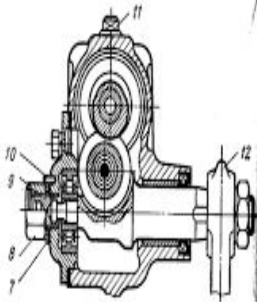
16.3. сурет. ГАЗ – 53 А автомобилінің рульдік механизмі.
