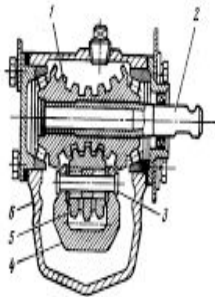
16.3. сурет. ГАЗ – 53 А автомобилінің рульдік механизмі.
