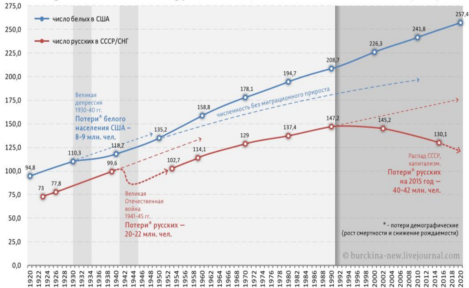
Сравнение численности русских в СССР/СНГ и белого населения США (млн.)
