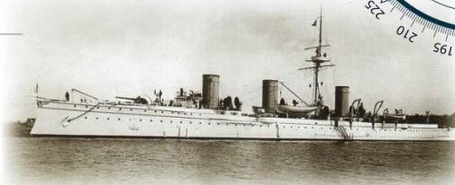
Бронеподъемный крейсер «Новик»
