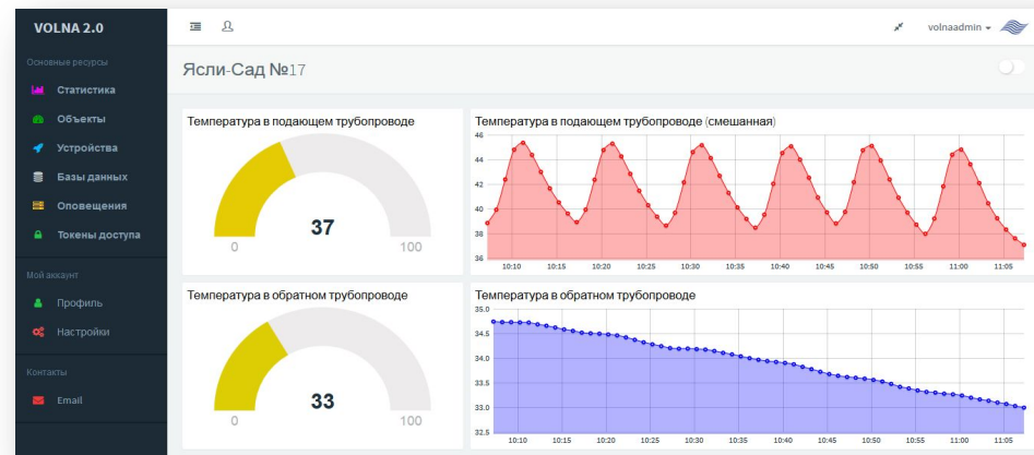
On-line диспетчеризация
