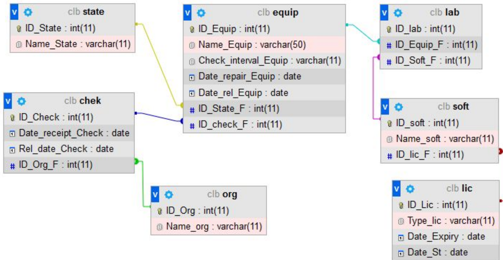
Рисунок 1 – модель базы данных “Laboratory”
