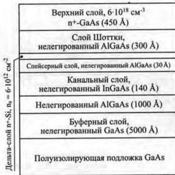
Структура псевдоморфного p-HEMT транзистора AlGaAs/InGaAs/GaAs
