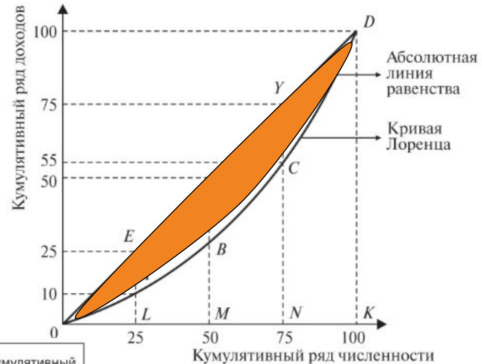
Рис 1. Кривая Лоренца
