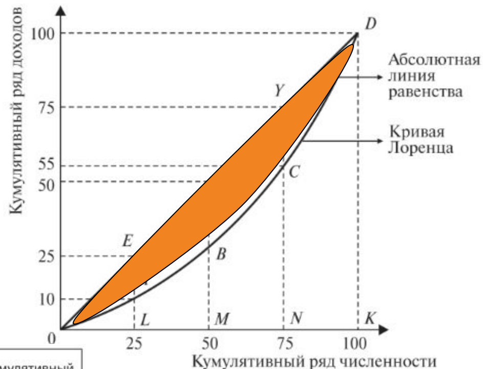
Рис 1. Кривая Лоренца
