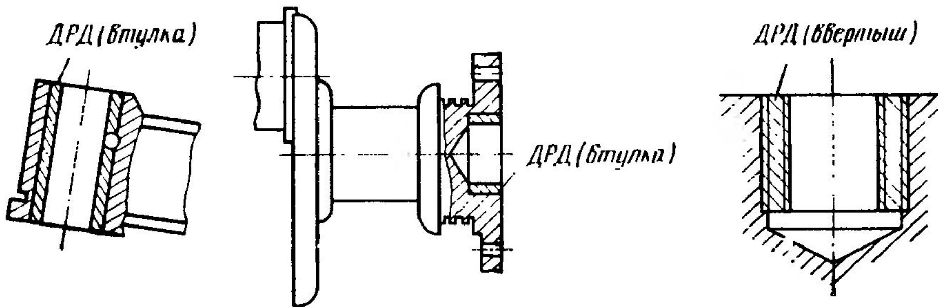
Рис. 13.2. Дополнительные ремонтные детали
