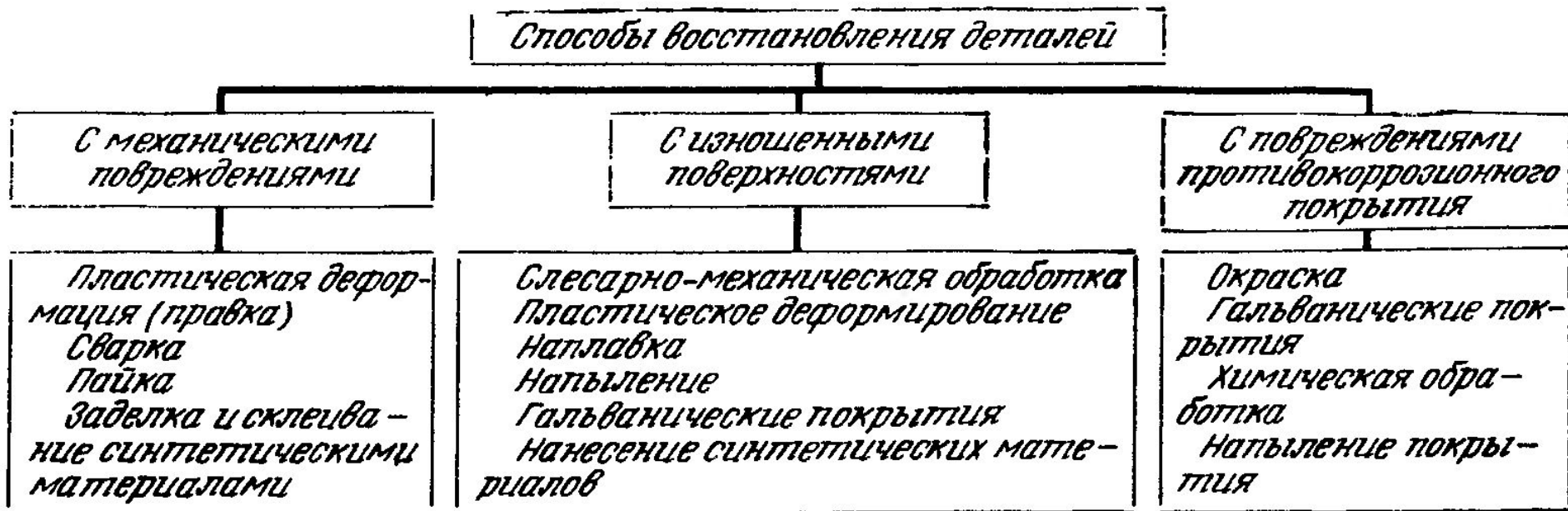
Рис. 12.1. Классификация способов восстановления деталей
