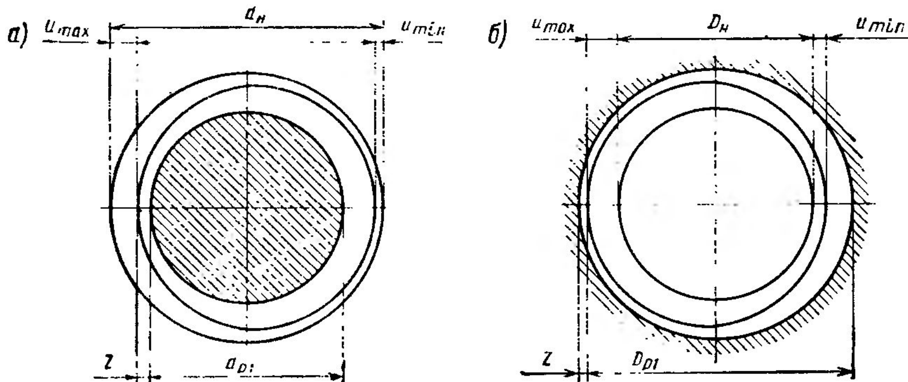
Рис. 13.1. Определение ремонтных размеров: а — для вала; б — для отверстия
