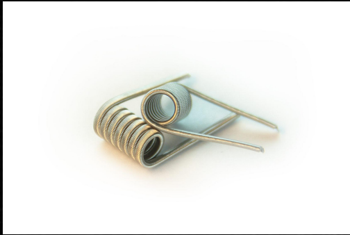
Fused Clapton \Omega=0,40 \text{ Ом} 2x0, 4Ni80+0, 1Ni80 7 витков на 3 мм оправу
