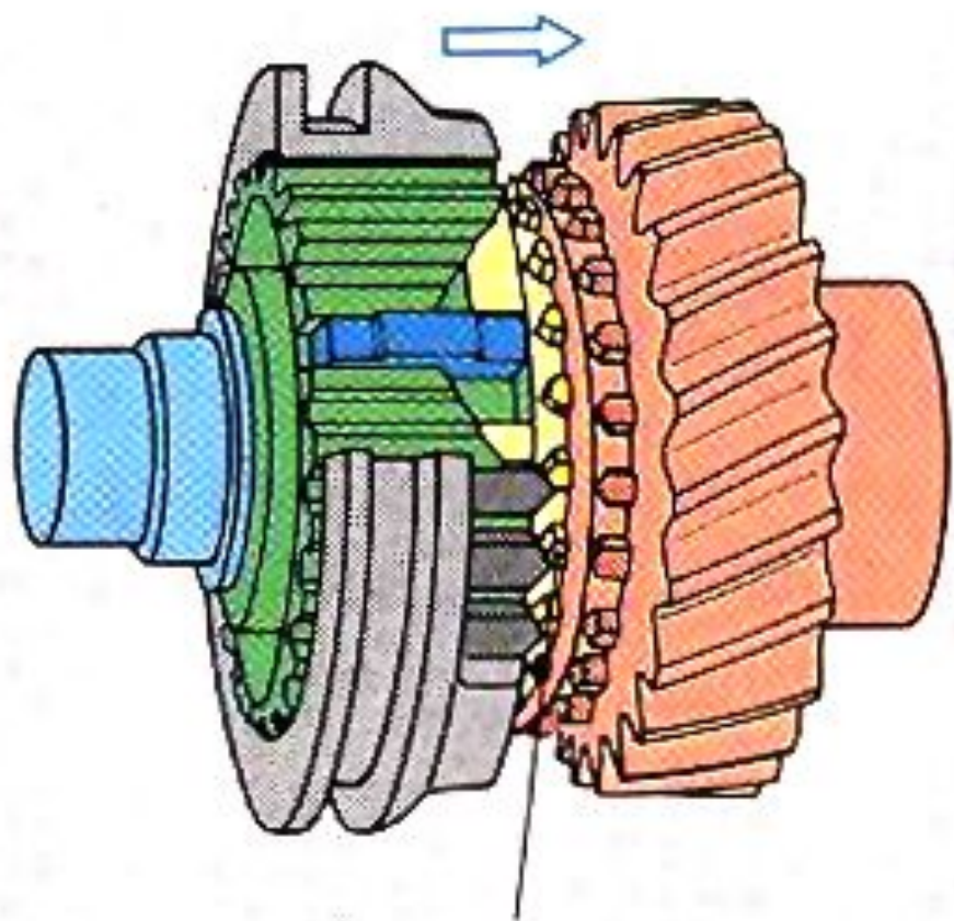
Sperrzähne auf Synchronring
