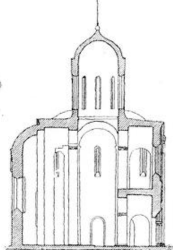
Продольный разрез
