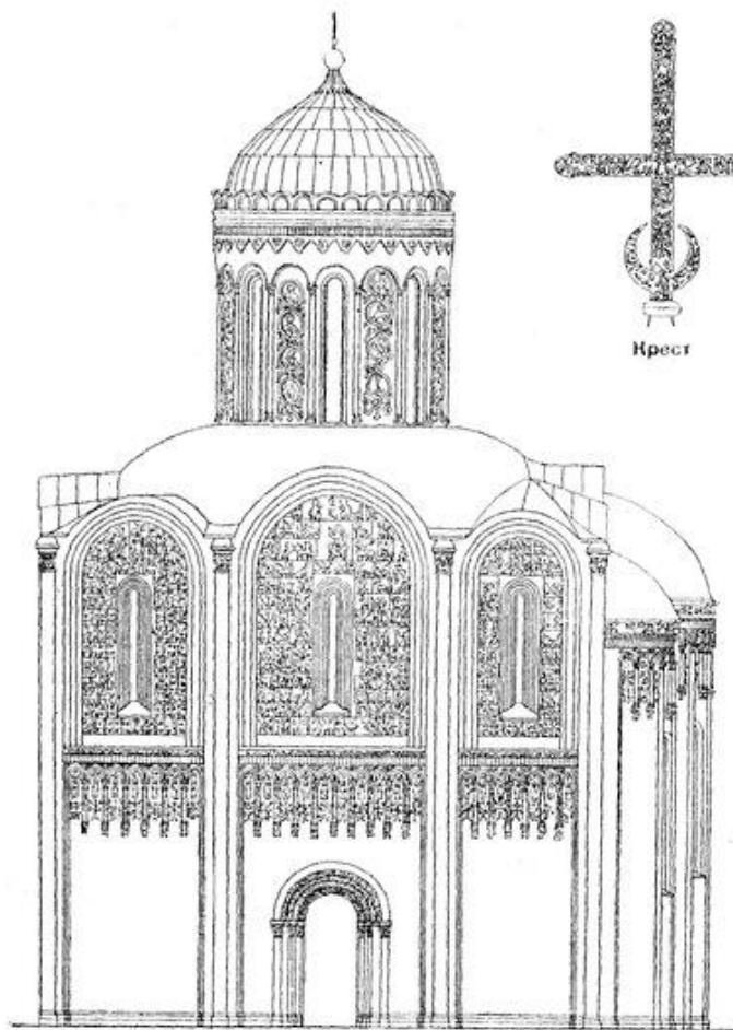
Южный фасад
