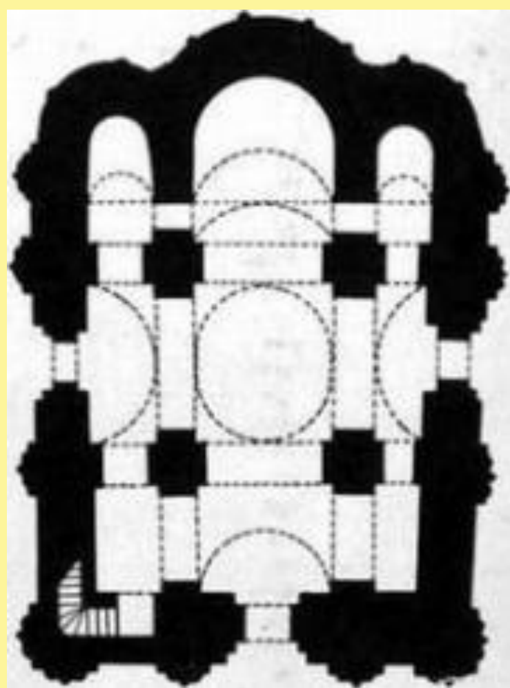
Пятницкая церковь. План-схема
