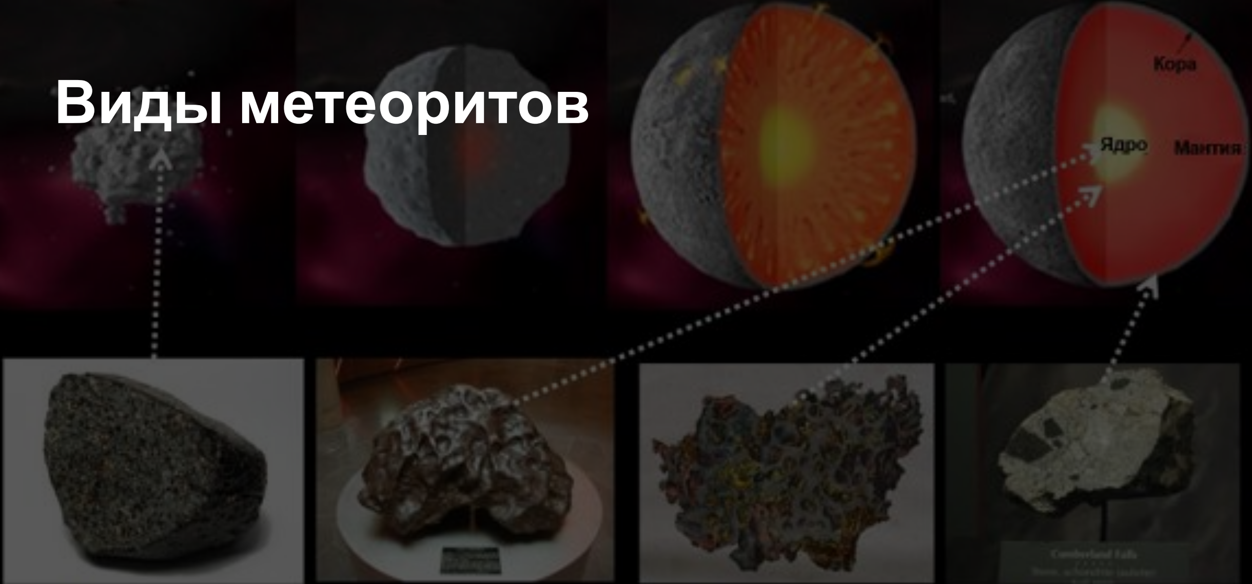
Хондриты
