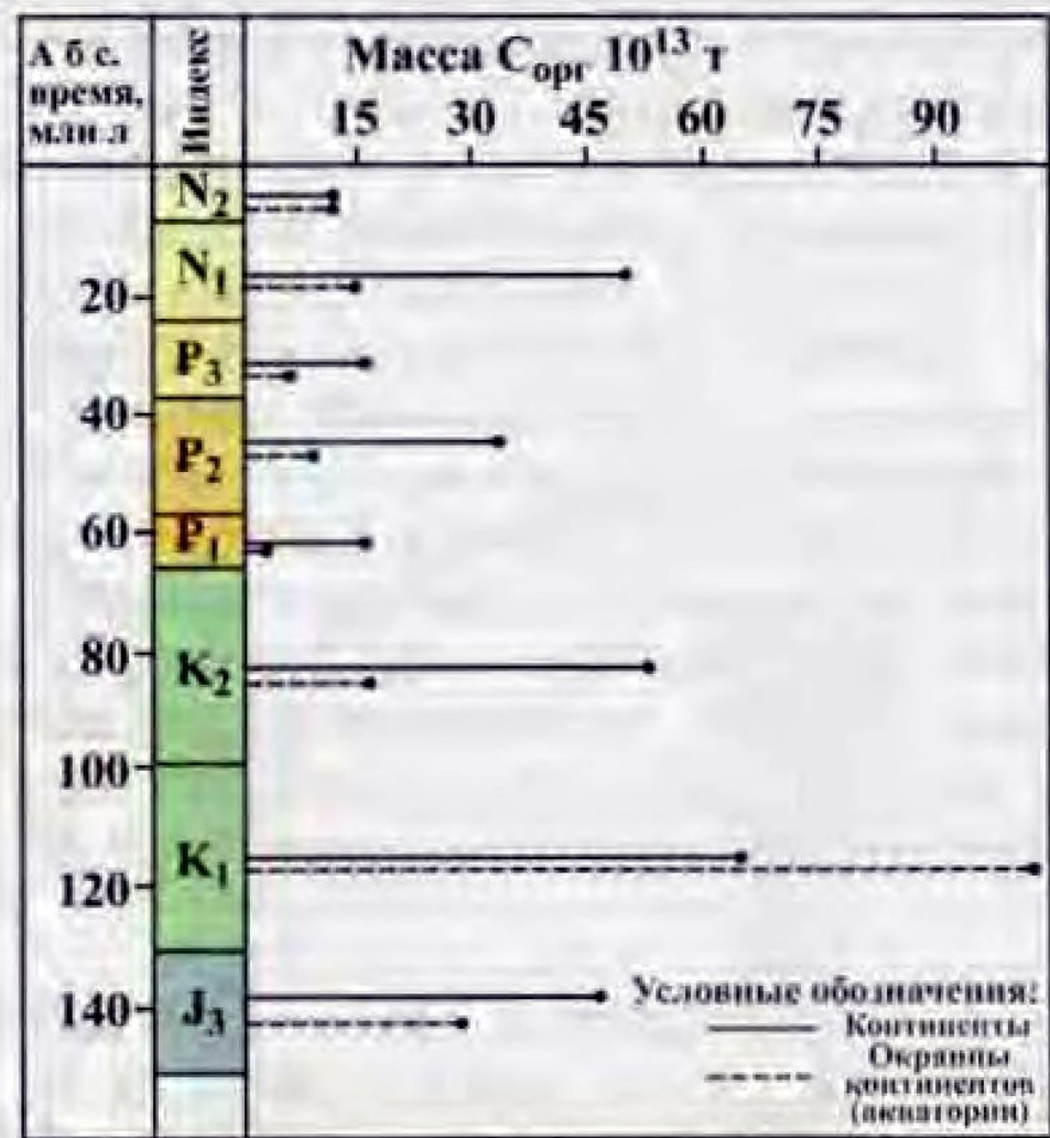
Рис. 3.12. Распределение массы органического углерода в породах и осадках континентов и океанов (по А.Б. Ронову, 1980)
