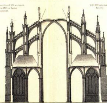
Quadratischer Querschiff mit Ansicht der Strebepfeiler u. Strebepfeiler.
