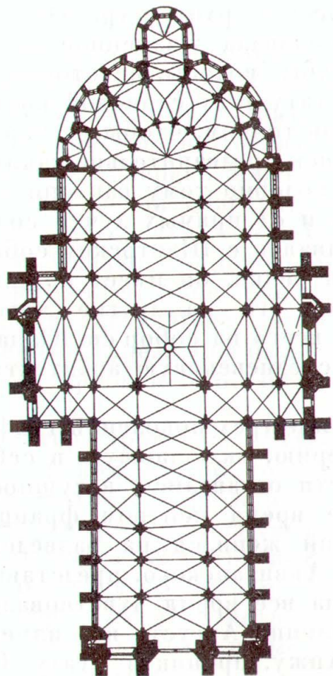
Собор в Амьене. План
