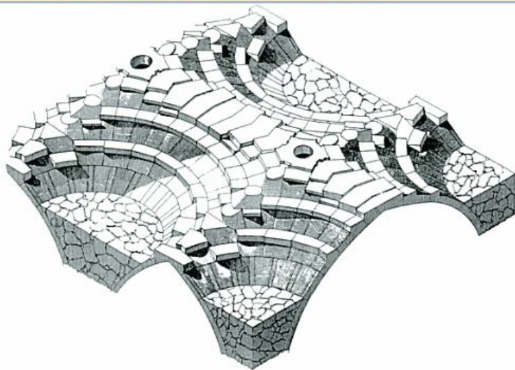
Figura 4.34 El coro posterior de la catedral de Peterborough (Willis, 1842)
