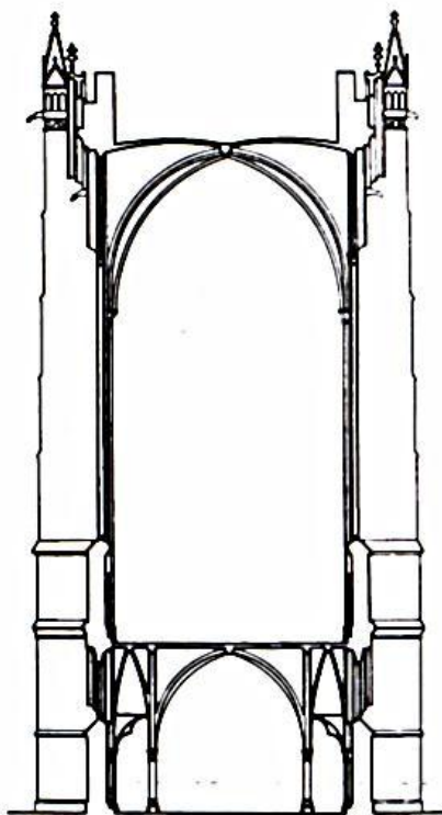
План. Поперечный разрез.
