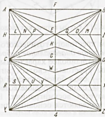
Рис. 218. Крестовые своды среднего нефа собора в Эксетере (Англия)
