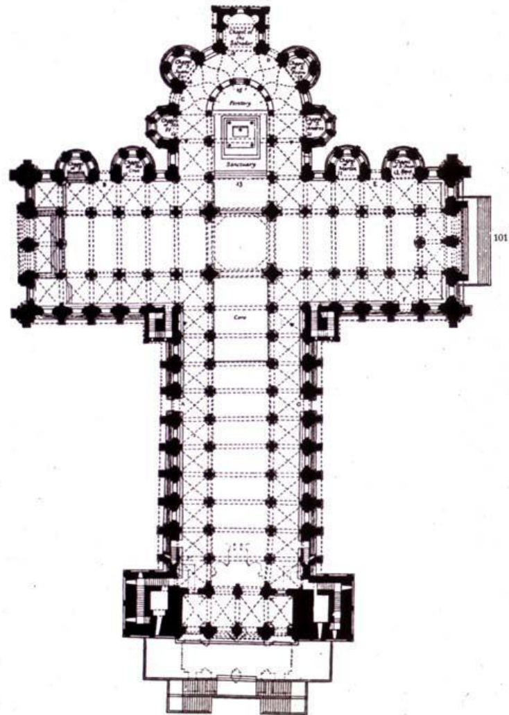
99-101 Compostela (Provinz Galicia), Kathedrale Santiago. Baubeginn 1077/78, Vollendung des romanischen Baus 1128. 99: Ansicht von der Südseite; 100: Längsschnitt durch den Kirchenraum; 101 Grundriß. (Sämtliche 1:500) — Nach Cosent
