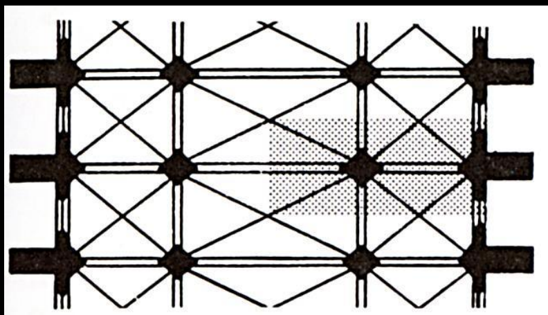
Травея с четырехчастными сводами в центральном нефе
