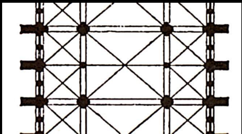
Травея с шестичастными сводами в центральном нефе
