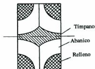
Figura 4.35 Vista en planta de un tramo de bóveda de abanico
