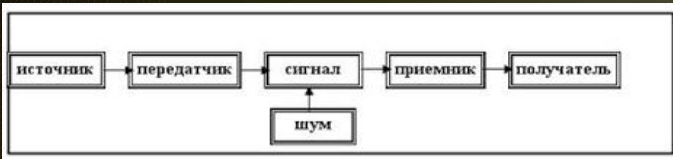
Шумовая модель коммуникации К. Шеннона - Уивера (1949)
