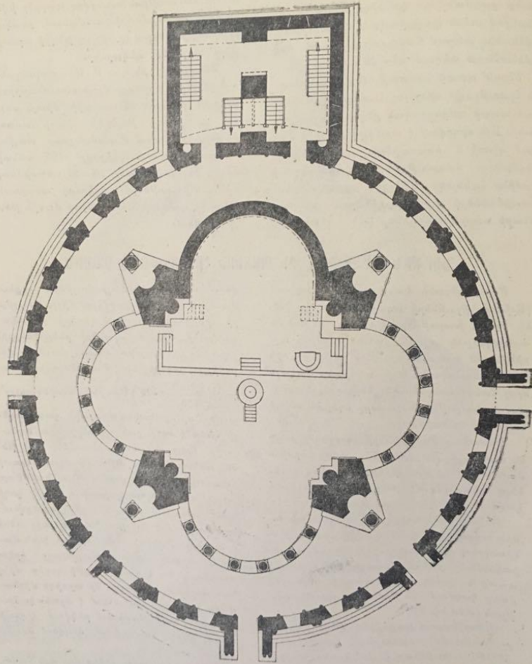
ՊՃ. 4. Զվարեացի առաջին ստաբնանի առաջին հարկարմնի հատակագիծ
