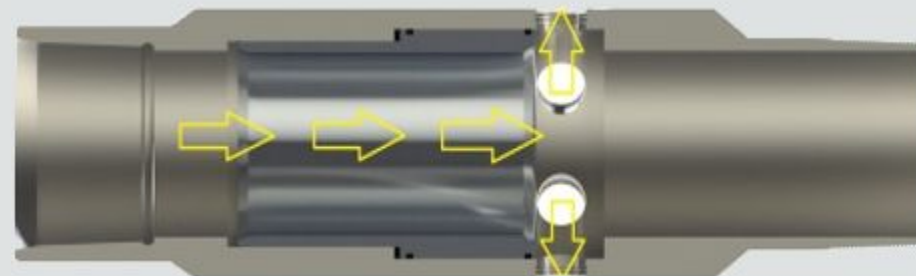
Б-ПХ-МГРП-Ш-114 открыт и готов к ГРП
