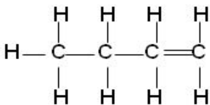
Олефин - бутилен-1
