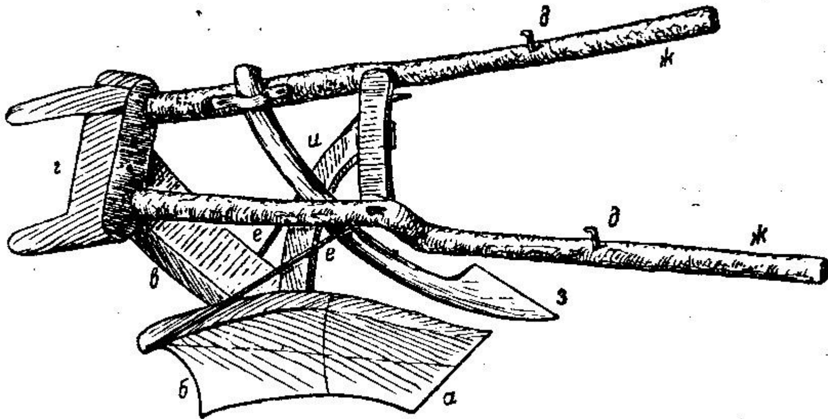
Соха «косуля» ; о — лемех; б — отвал; в — плотина; г — рогаль; д — крючки для пристяжки лошади; е — подвой железные; ж — оглобли; а — отрез; и — стужень (грядиль)
