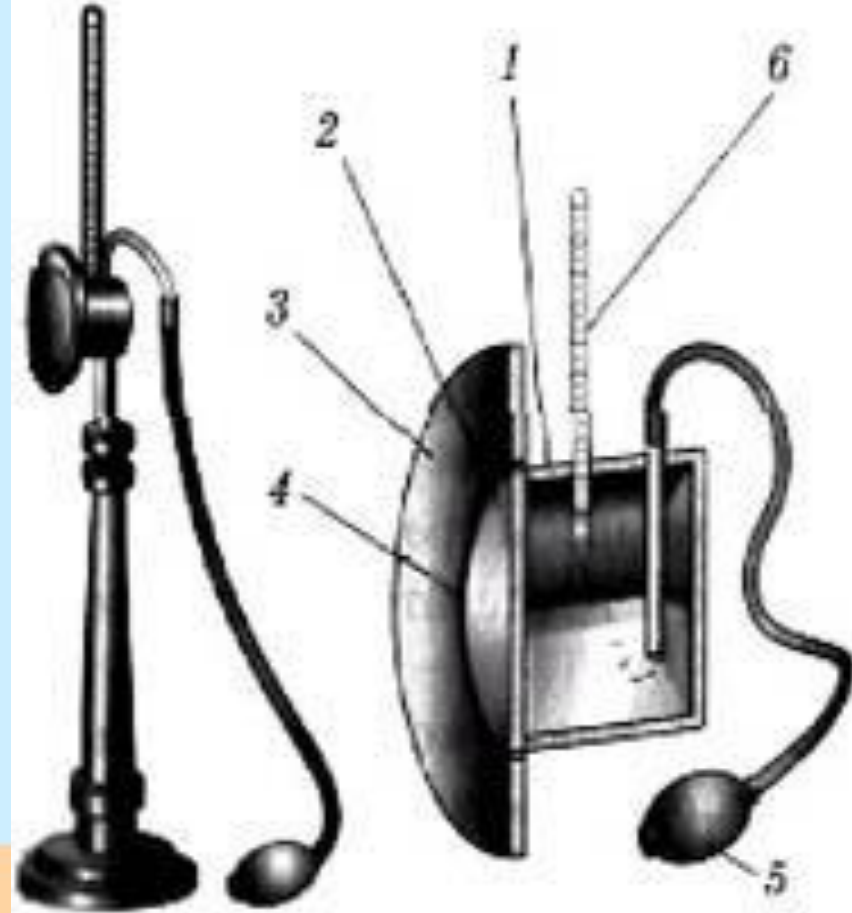
Гигрометр конденсационный
