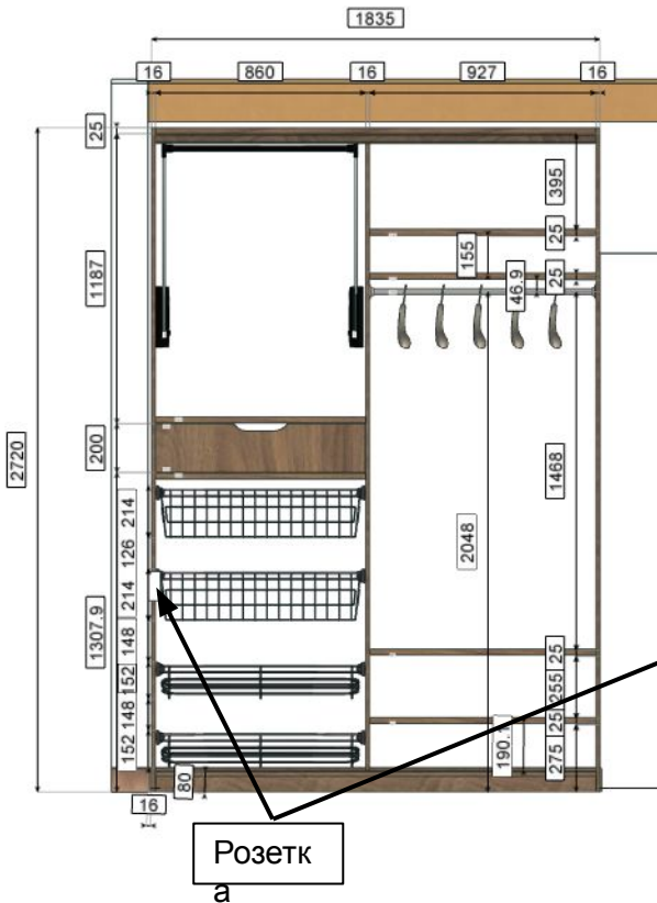
Фронтальный
