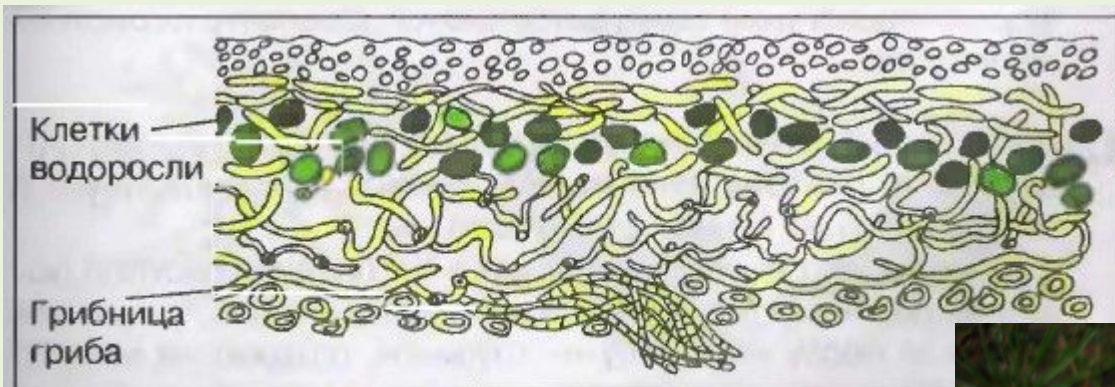
43. Строение лишайников
