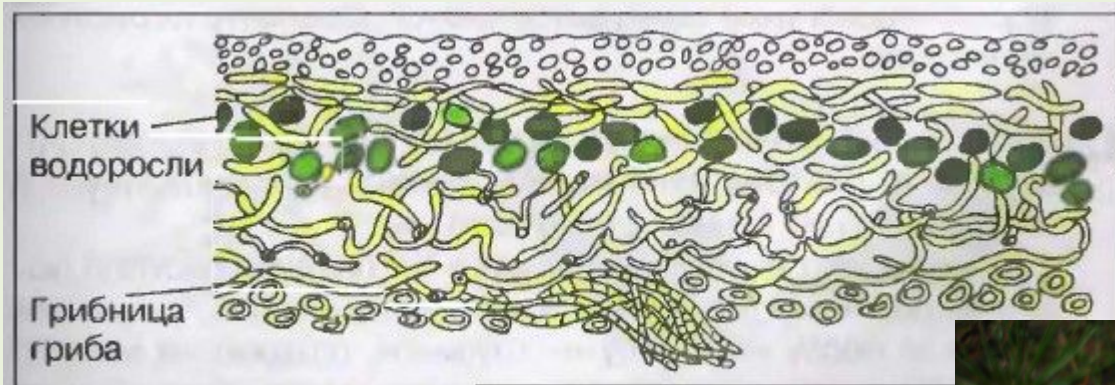
43. Строение лишайников
