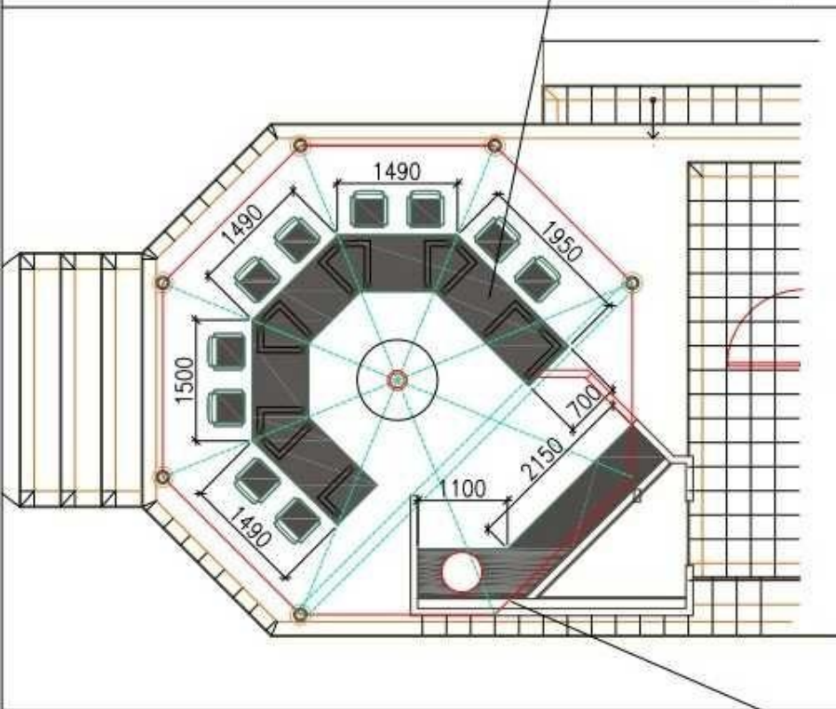
ПЛАН БЕСЕДКИ С РАССТАНОВКОЙ МЕБЕЛИ
