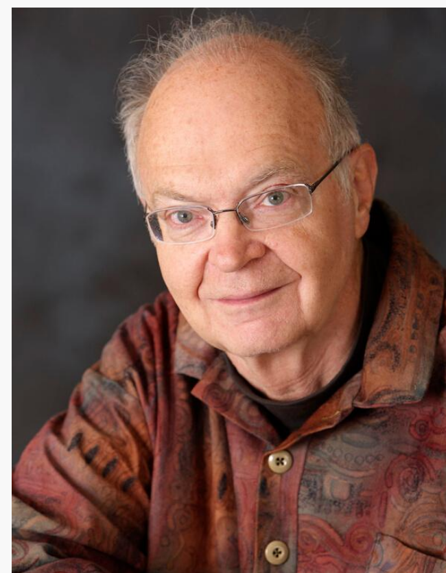
Дональд Кнут
