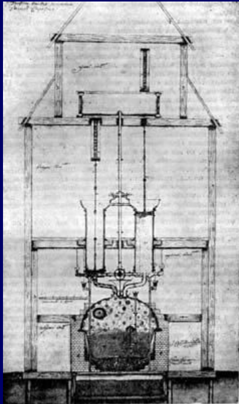
Поперечный разрез первой паровой заводской машины, изобретенной И. И. Ползуновым в 1763 году
