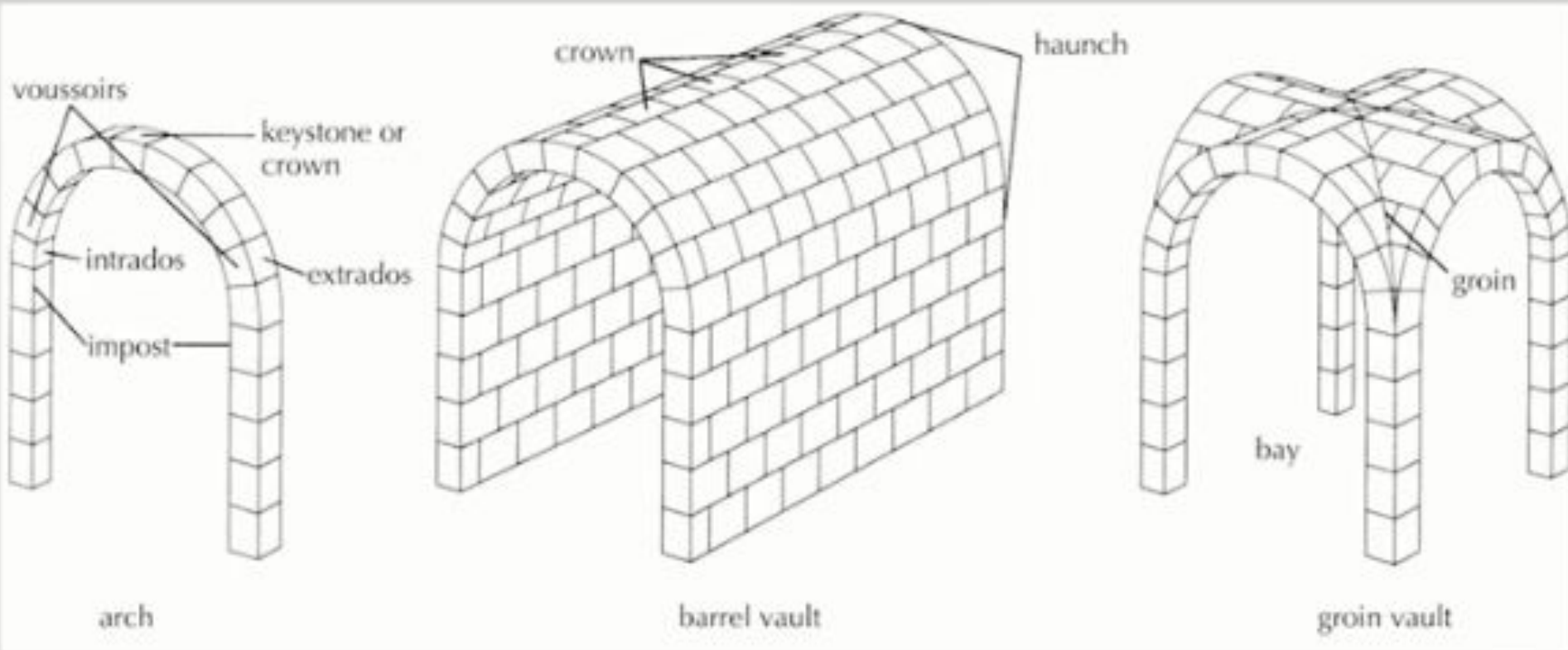
Арка, цилиндрический свод и крестовый свод.
