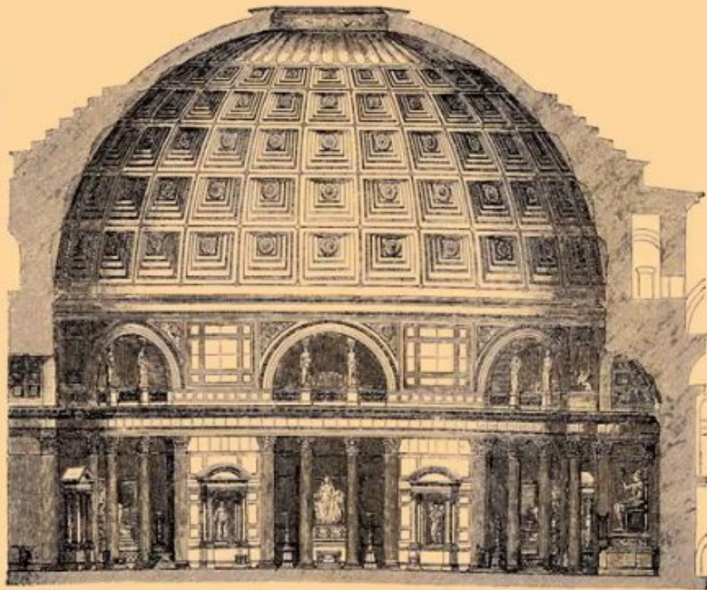
Внутренность в древности, по реставрации Адлера (Разрез)
