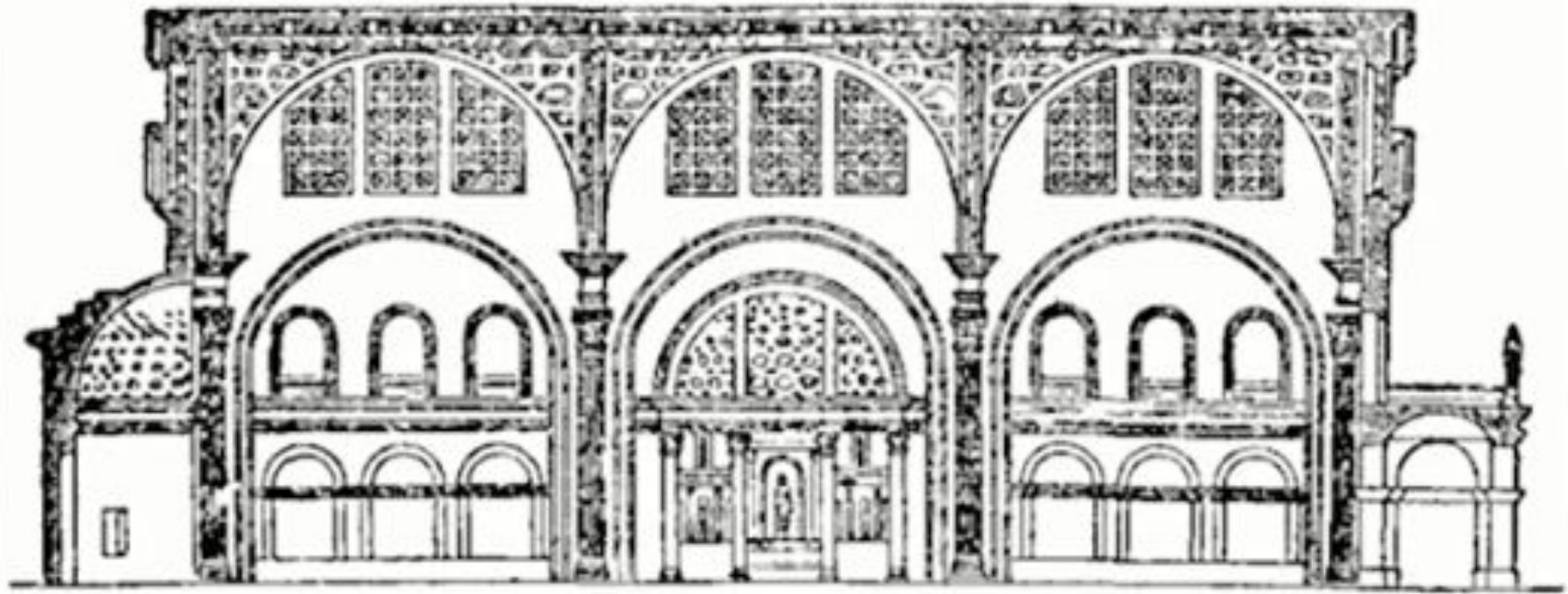
*Базлика Максенция-Константина в Риме. Реконструкция. 312 г.
