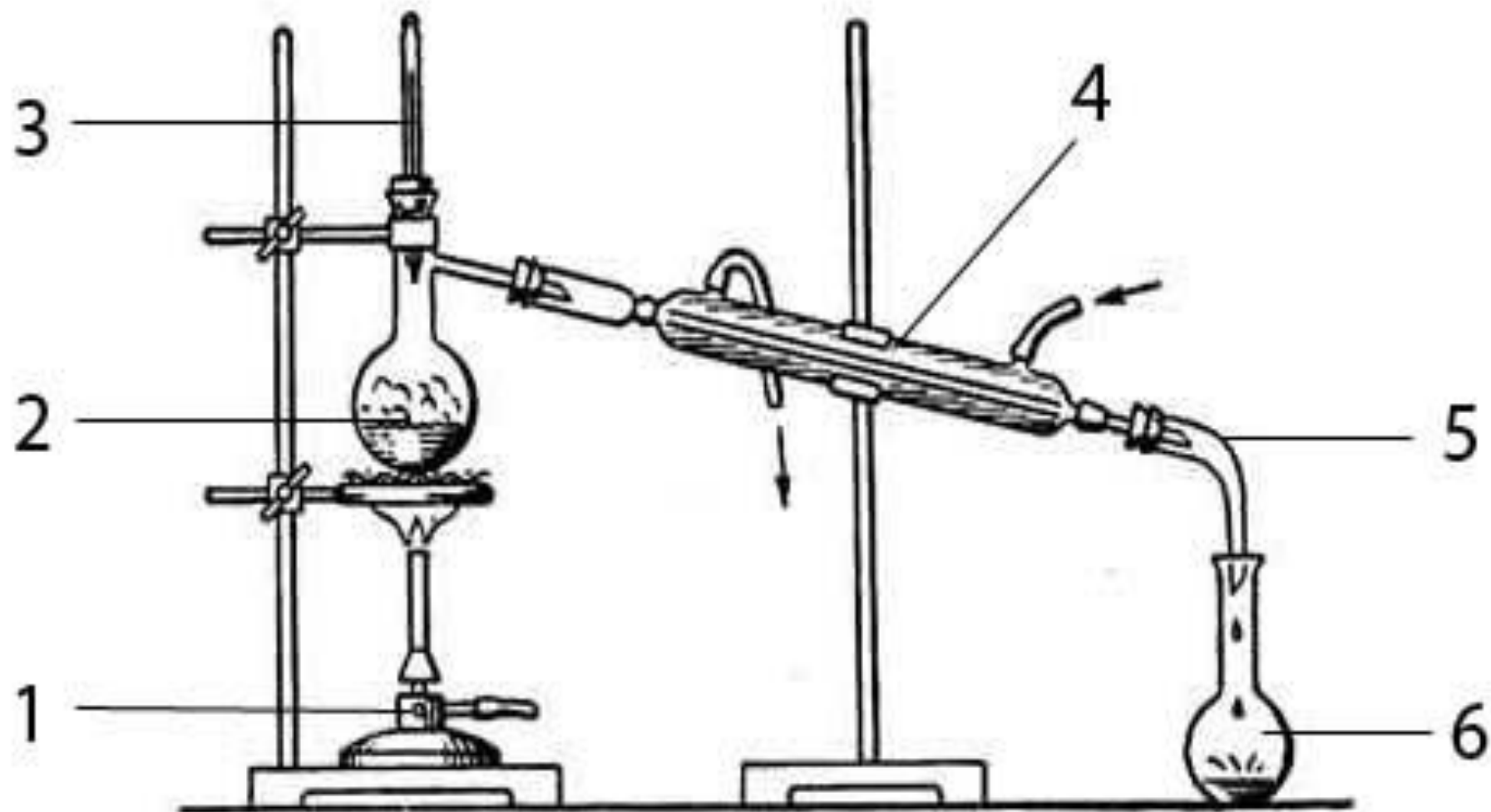
Прибор для перегонки жидкостей
