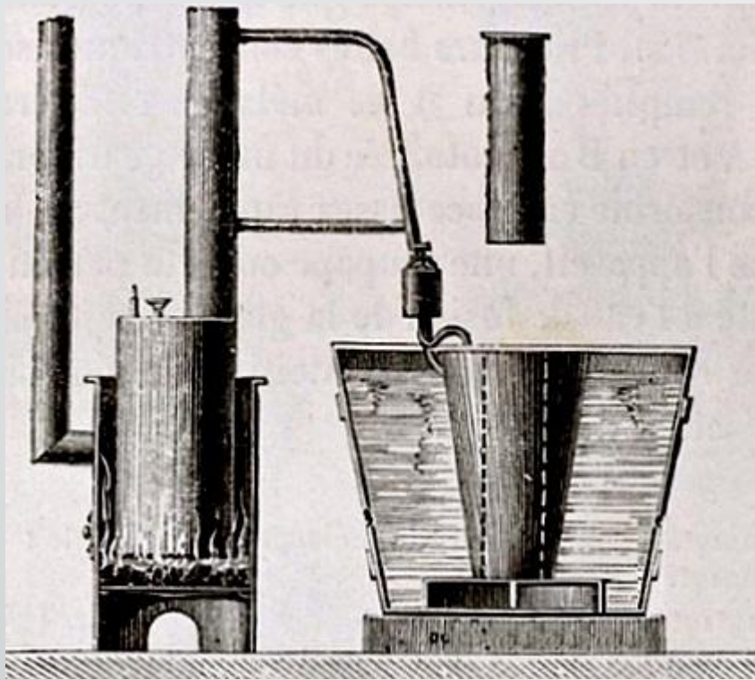
Абсорбційна холодильна машина Фердинанда Карре
