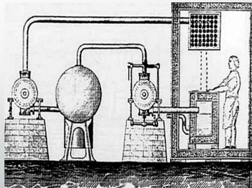
Фердинанд Карре, перша холодильна машина
